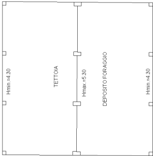
FABBRICATO "C" PIANO TERRA
