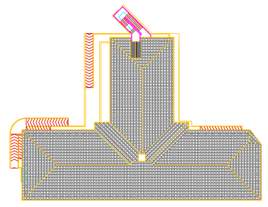
PIANO COPERTURA
