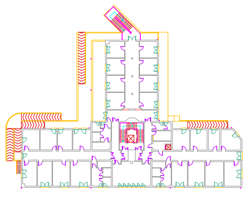
PIANO PRIMO
